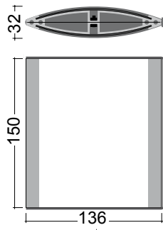
2 FLÜGELSCHILD 84201G
