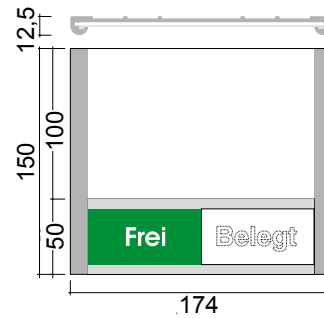
3 TÜRSCHILD, TYP B MIT MANUELLER FREI/BELEGT-ANZEIGE 84129G FREI/BESETZT-ANZEIGE 84102G
