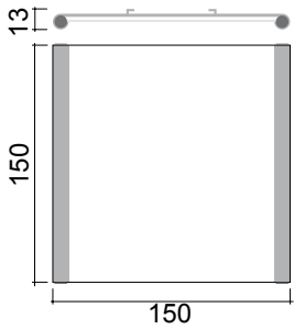
1 TÜRSCHILD, TYP A, VOLLRUNDPROFIL 84100G
