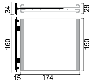
6 FLÜGELSCHILD, TYP B 84104G
