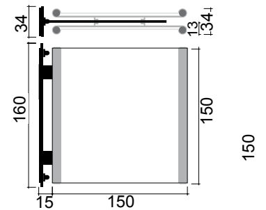
6 FLÜGELSCHILD, TYP A 84103G
