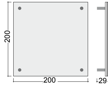
3 TÜRSCHILD 200 x 200 mm 84174G
