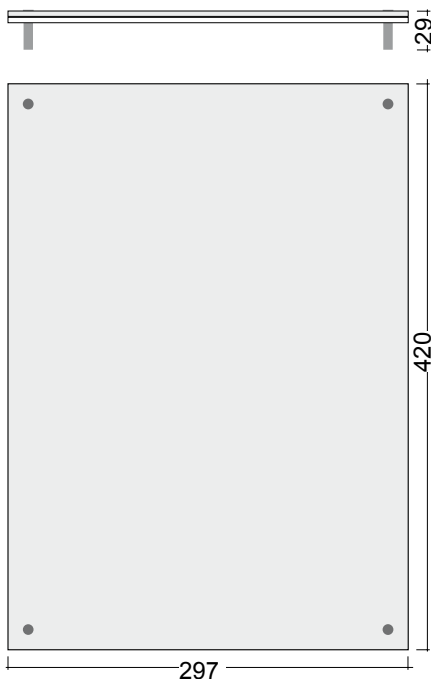
6 WANDSCHILD A3 HF 297 x 420 mm 84153G
