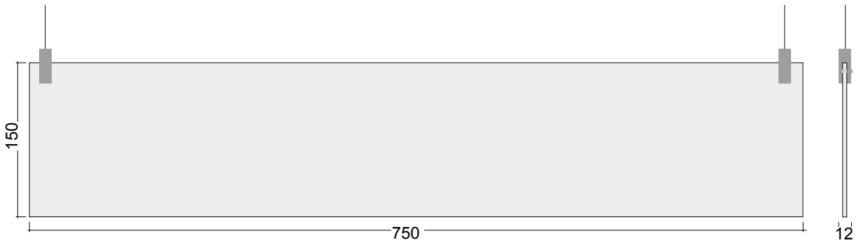
9 DECKENPANEEL 750 x 150 mm 84157G
